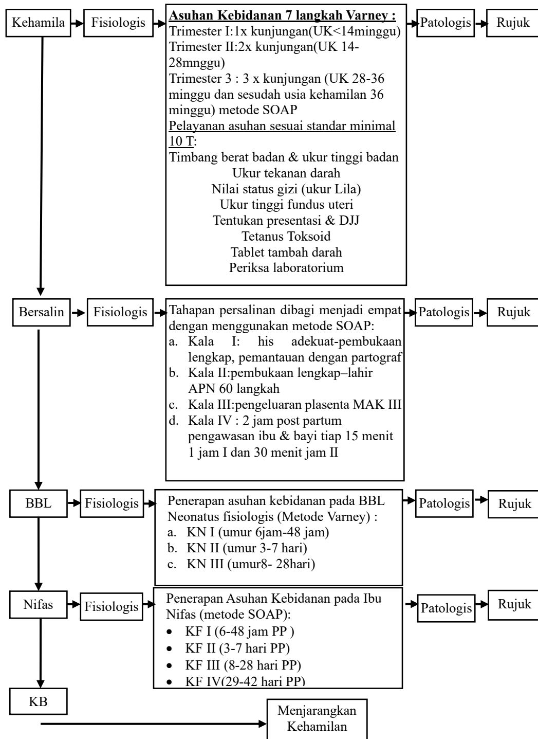
Gambar 1 Kerangka Pikir
