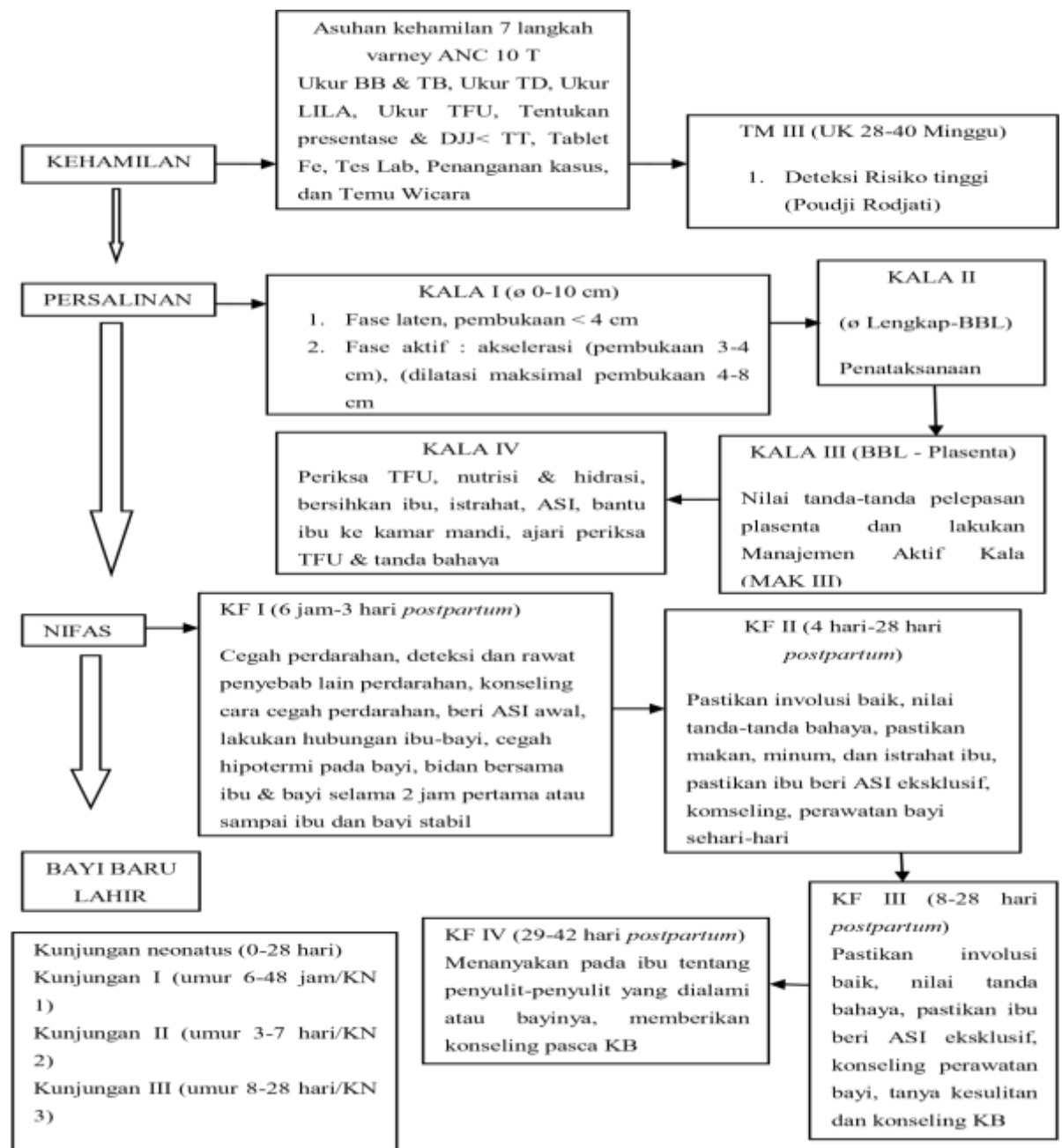
Gambar 2. 1 Kerangka pikir
