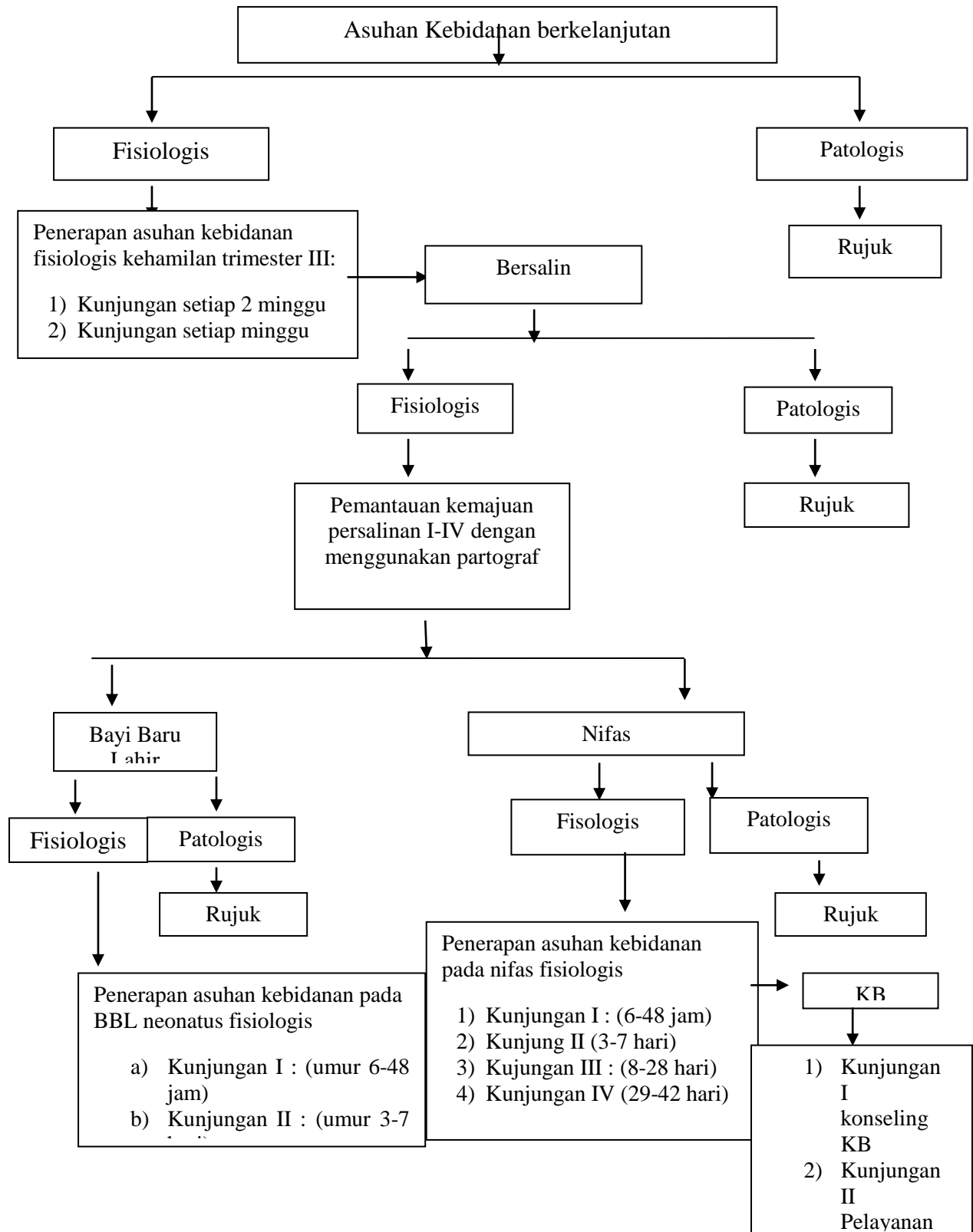
Gambar 2.1 kerangka Pikir
